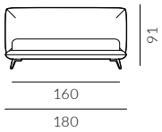
Blow, szerokość materaca 160 cm, wysokość wezgłowia 91 cm, tkanina Kirkby Design Smooth III K5228/62 Combat, kedra Sorensen Dunes Cognac, noga M8-145 lakierowana proszkowo w kolorze brązowym
